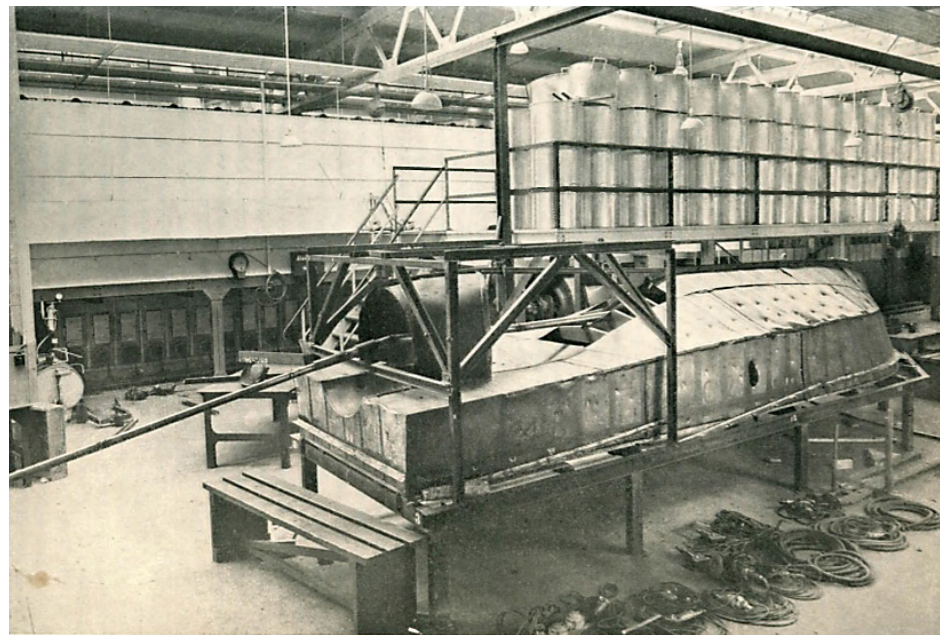
Fra en Sabotage i Fordfabrikerne i Sydhavnen i København, hvor et hold sabotører trængte ind og ødelagde to hurtigmotorbåde, som skulle afleveres til tyskerne et par dage efter. På billedet ses nogle af de huller, som sabotørerne med svejseapparater borede i bådene. Medens man var i gang med dette arbejde, dukkede en tysk militærdelegation op for at bese bådene. De modtoges af maskinpistolbevæbnede sabotører, som afvæbnede dem, hvorpå de fik lov til at overvære resten af Sabotagen.
