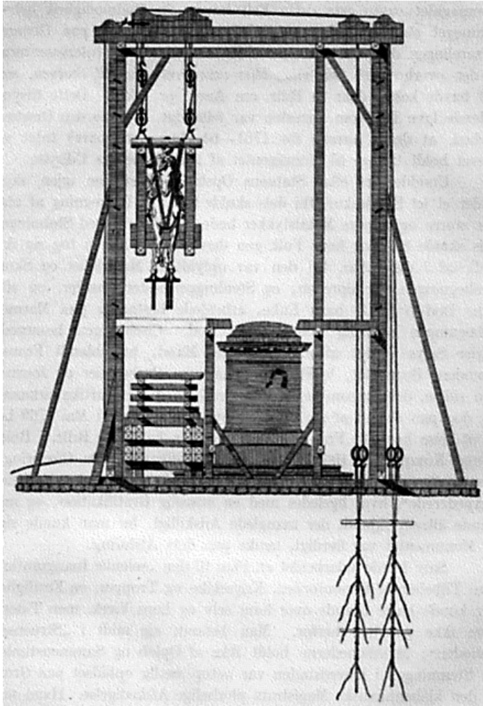
Maskineriet ved Rytterstatuens Opstilling.
