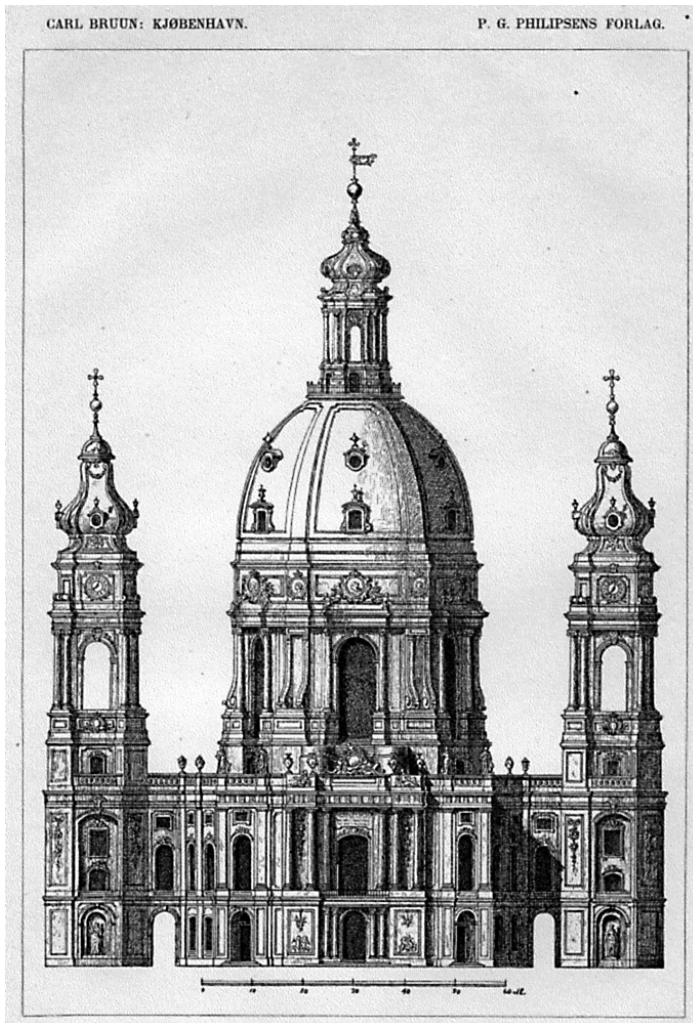
Eigtveds ændrede udkast til Frederikskirken, dat. 10de April 1754. (Efter en i 1892 til Rigsarkivet afleveret Tegning.)
